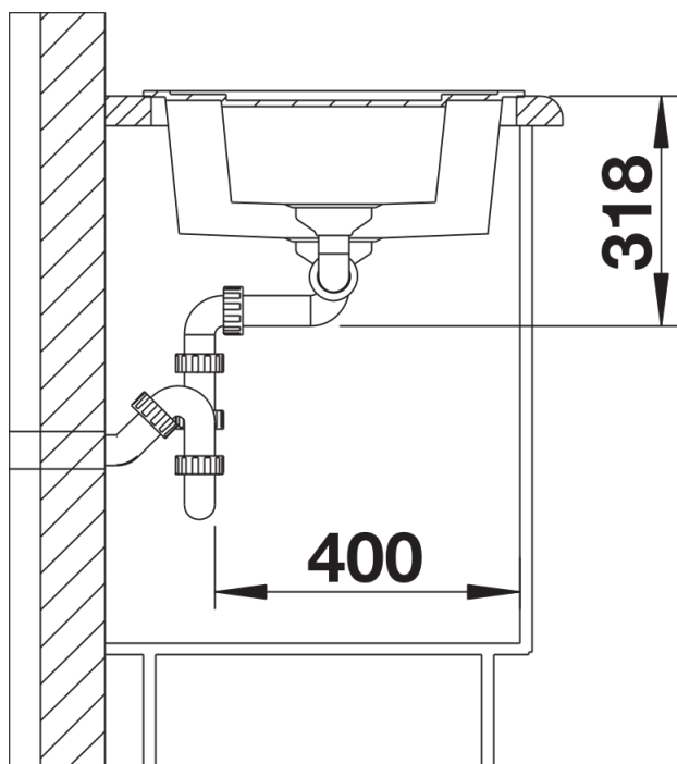
Seitenansicht
