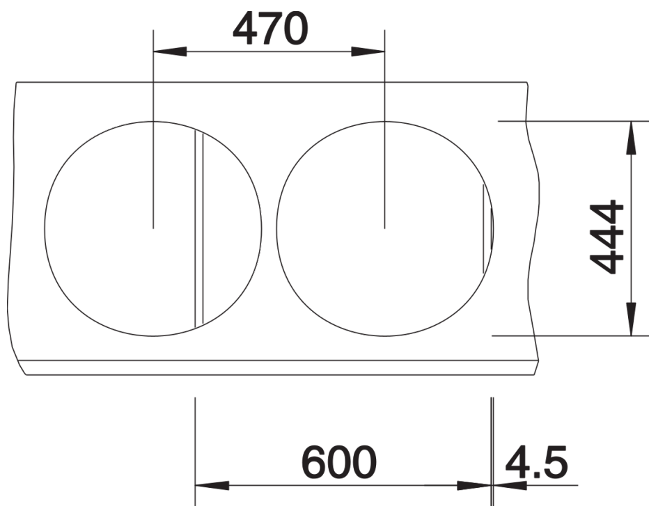
Ausschnitt
