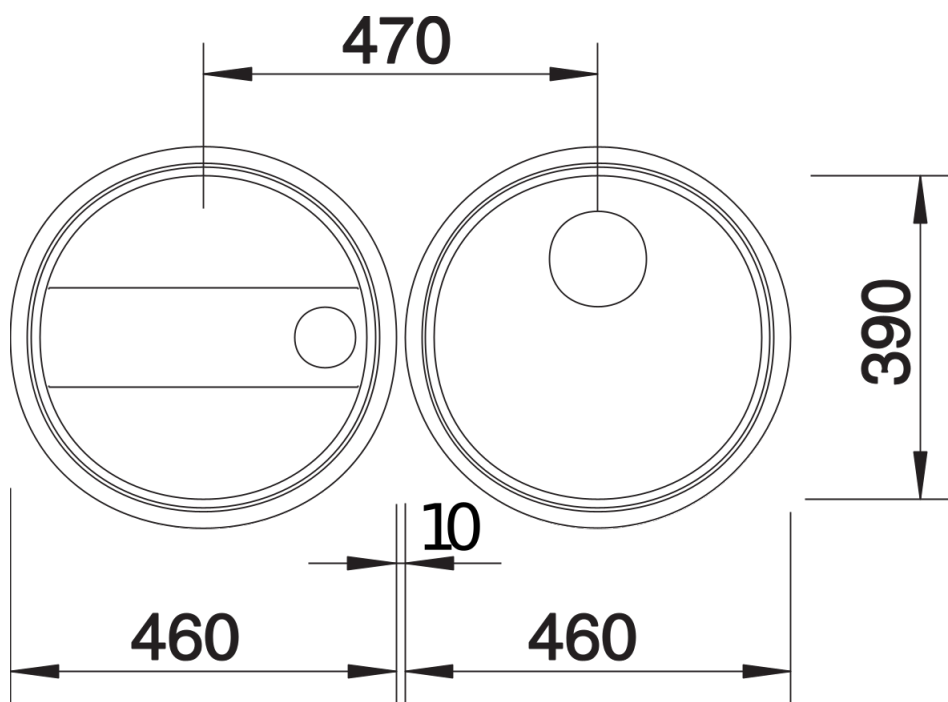
Aufsicht
