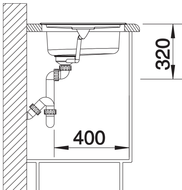
Seitenansicht
