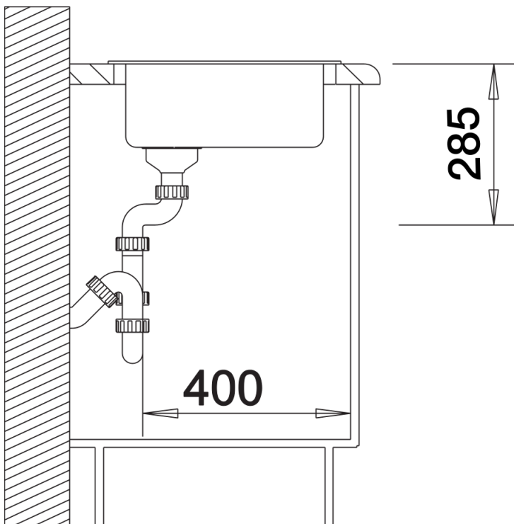
Seitenansicht
