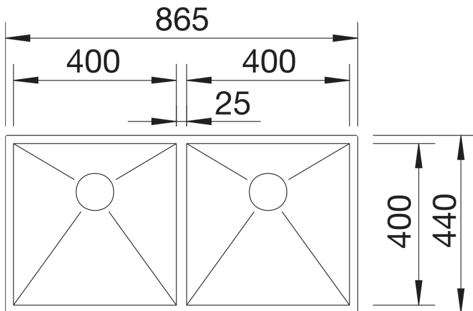
Aufsicht
