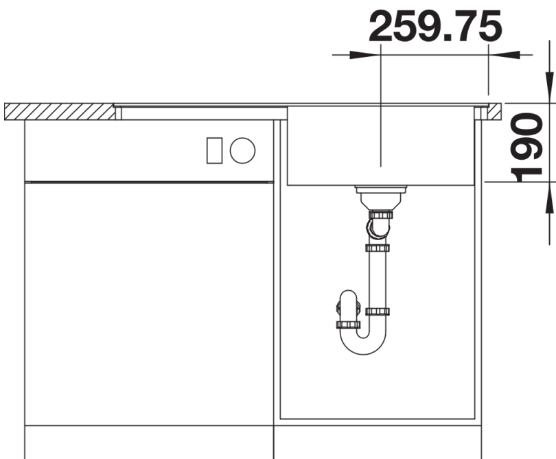
Frontansicht
