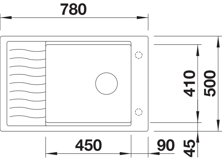
俯视图
