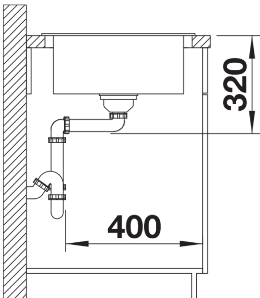
侧视图
