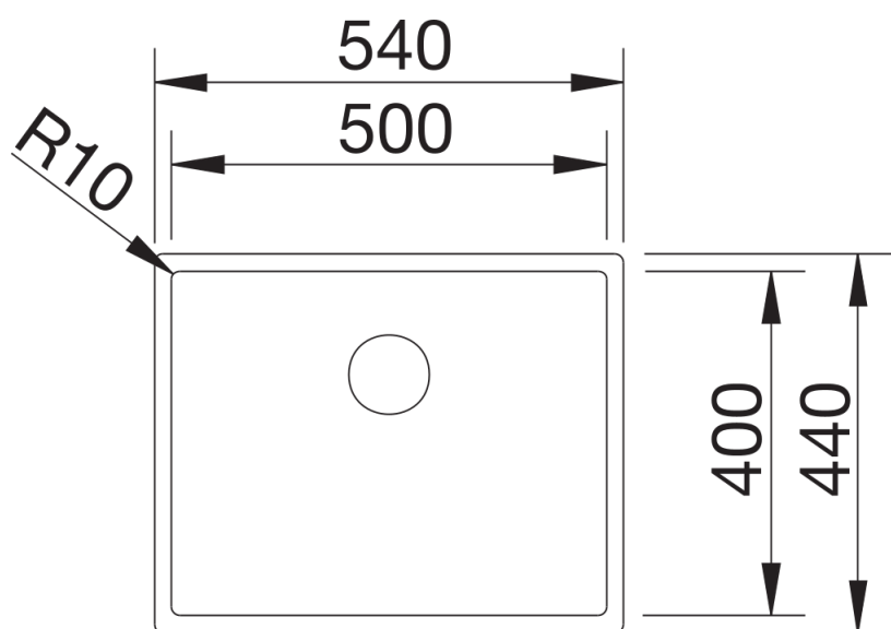
俯视图
