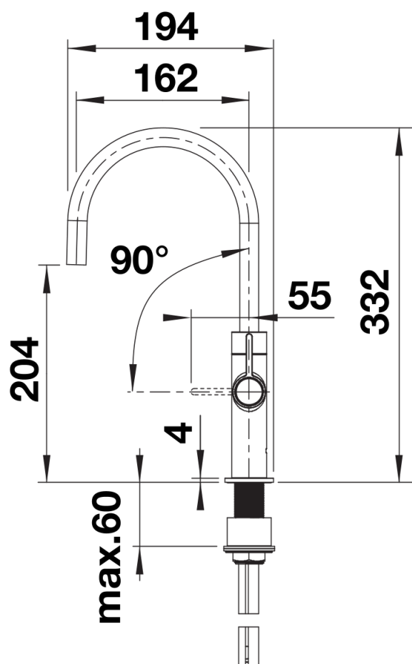
侧视图
