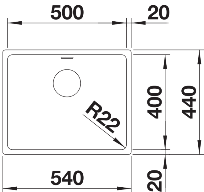
俯视图
