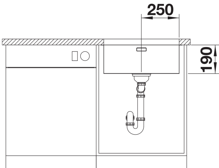
正视图
