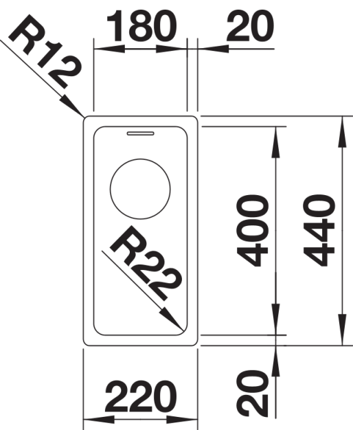
俯视图
