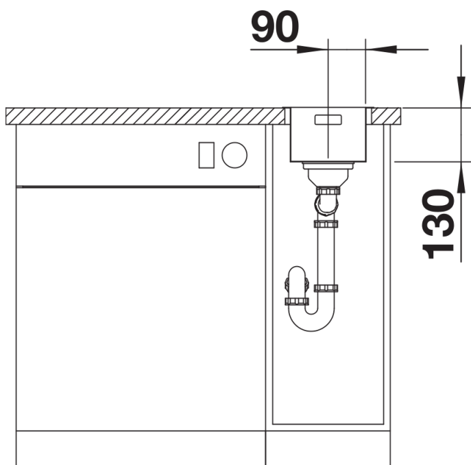
正视图
