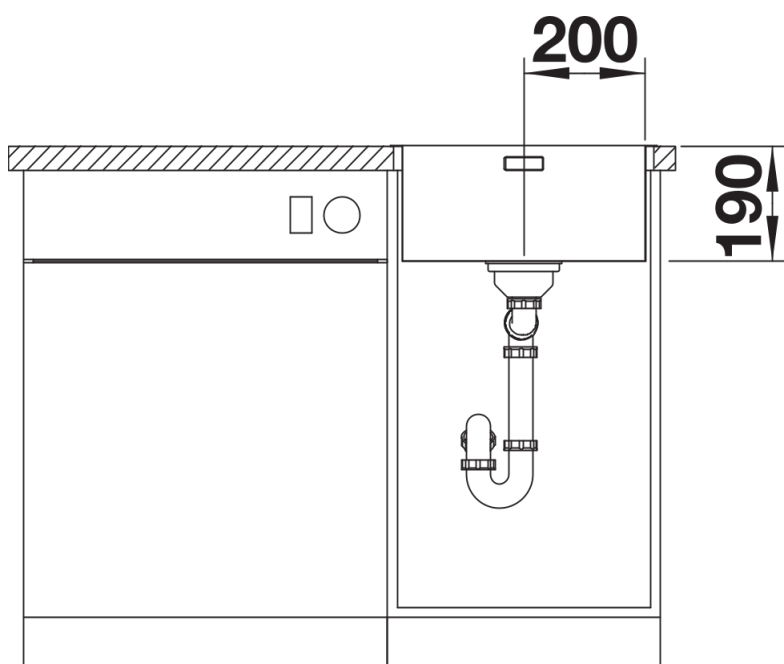
正视图
