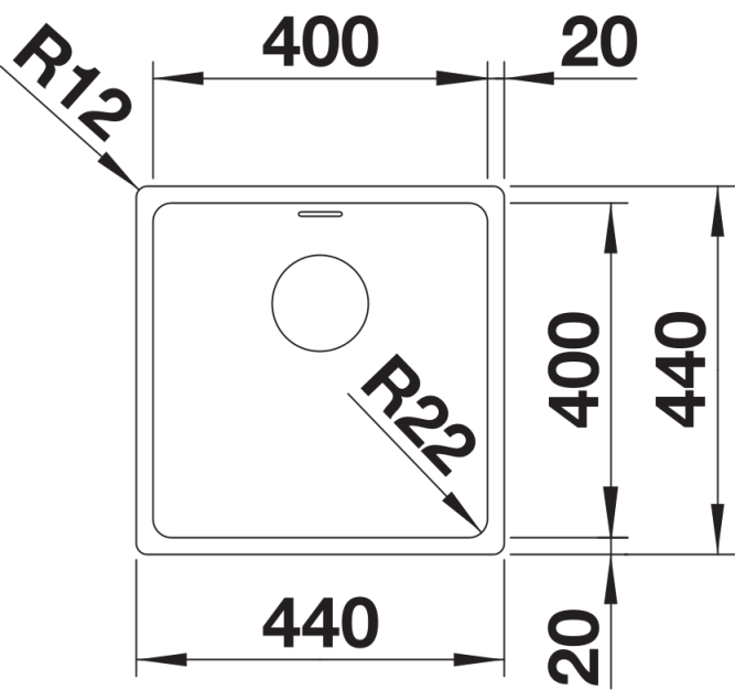
俯视图
