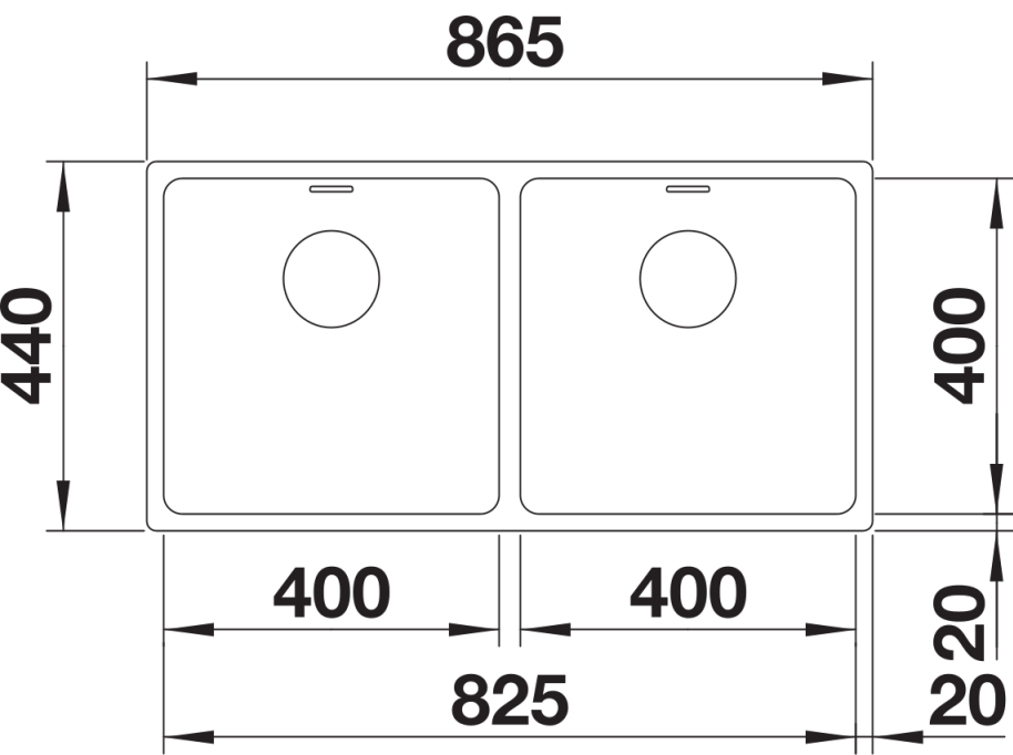
俯视图
