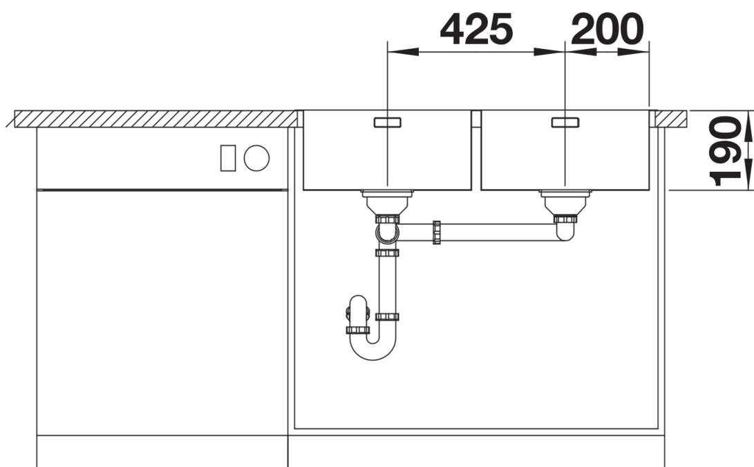
正视图
