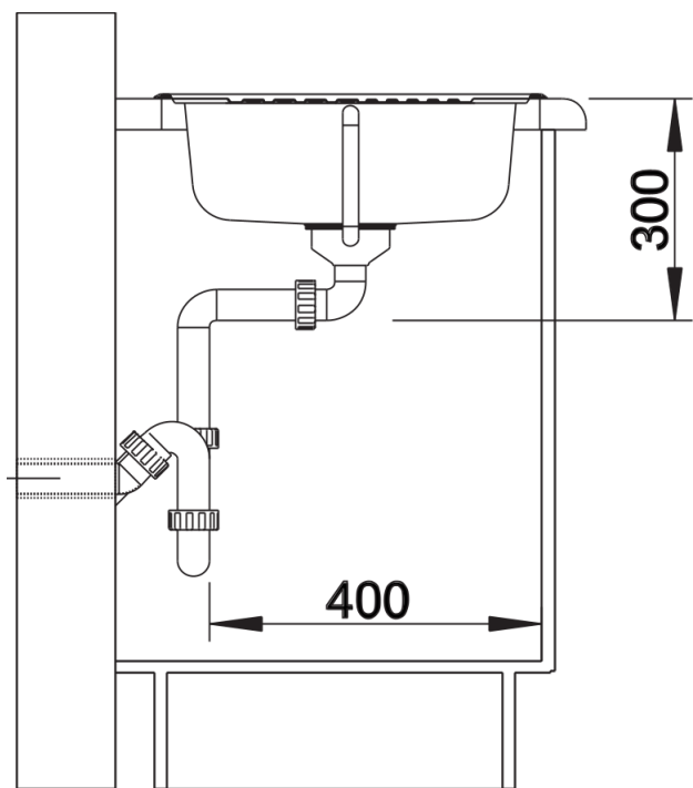
侧视图
