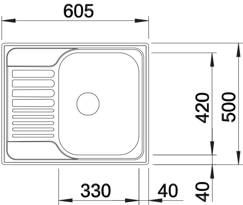
俯视图
