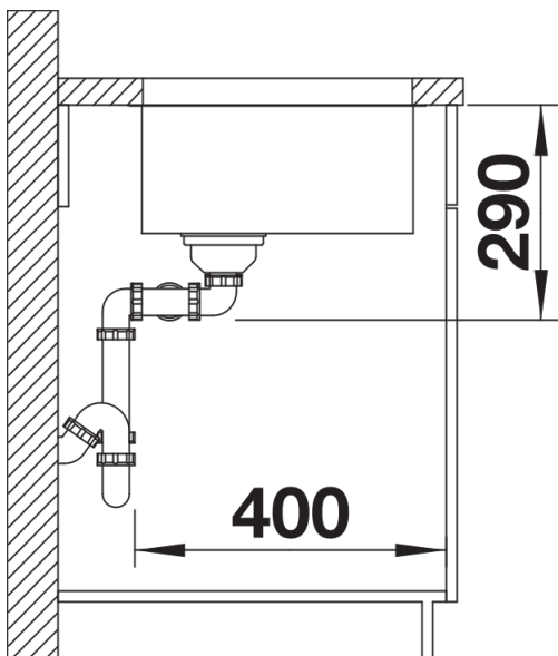
侧视图
