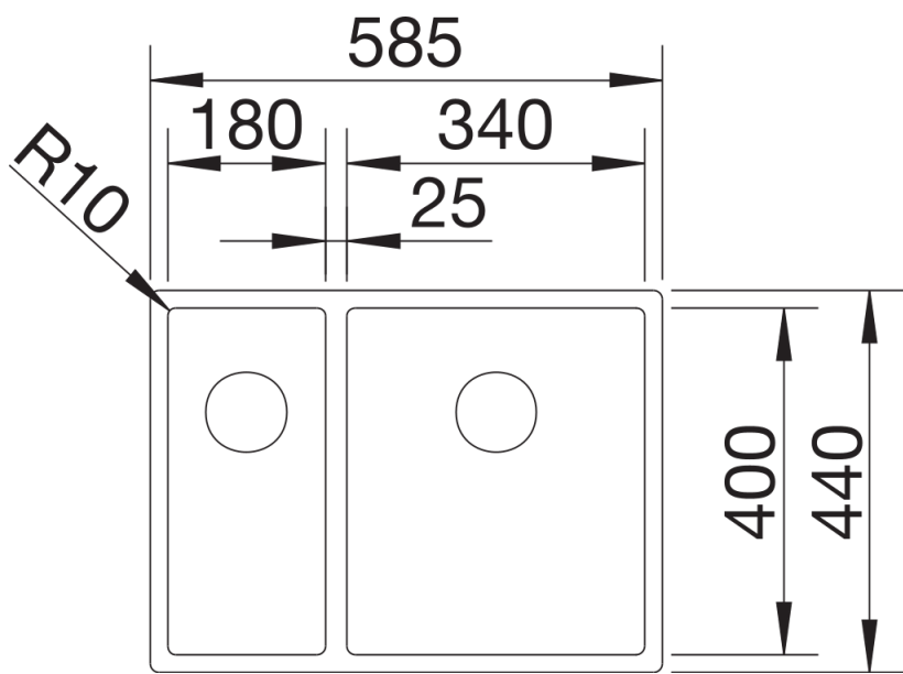
俯视图
