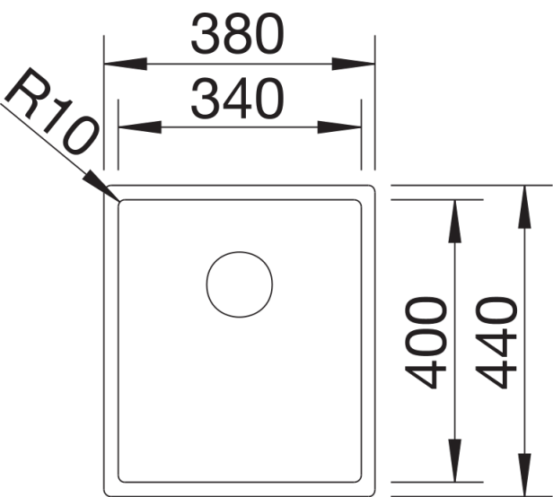
俯视图
