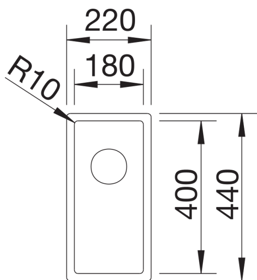
俯视图
