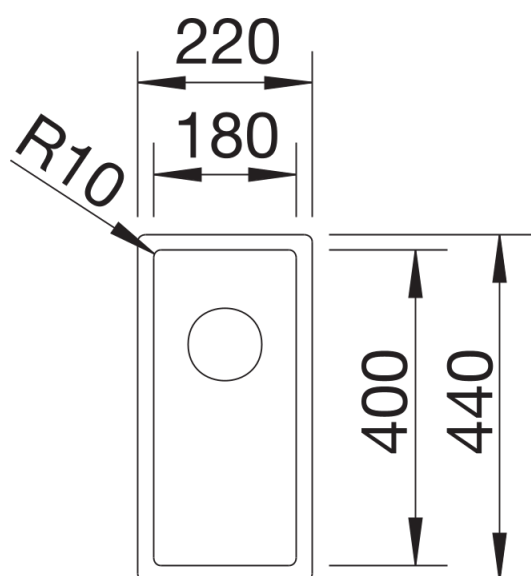
俯视图
