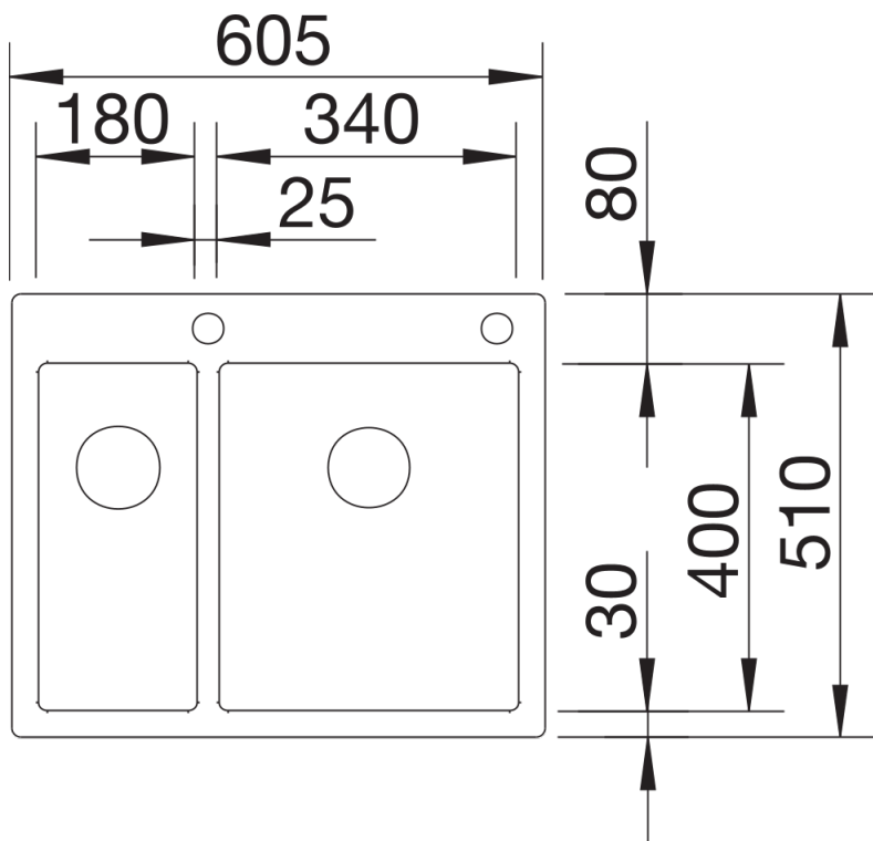
俯视图
