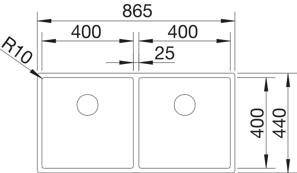
俯视图
