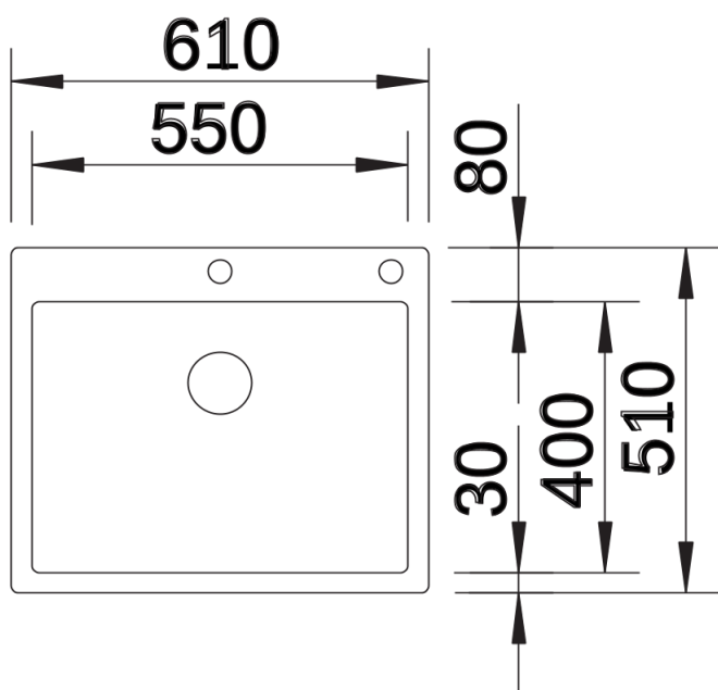
俯视图
