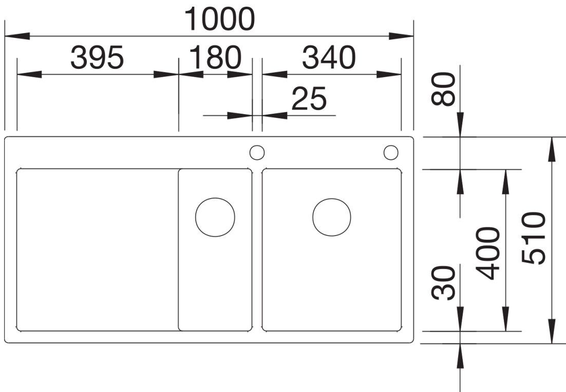
俯视图
