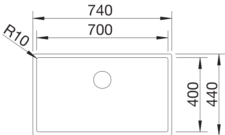
俯视图
