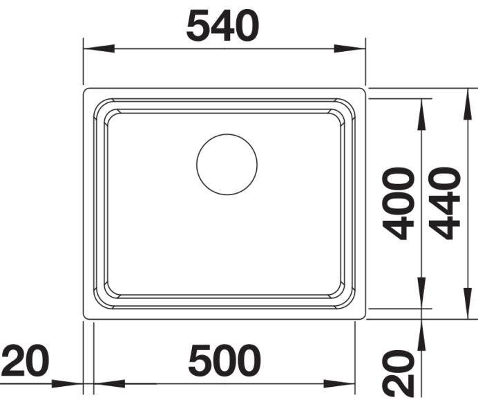
俯视图
