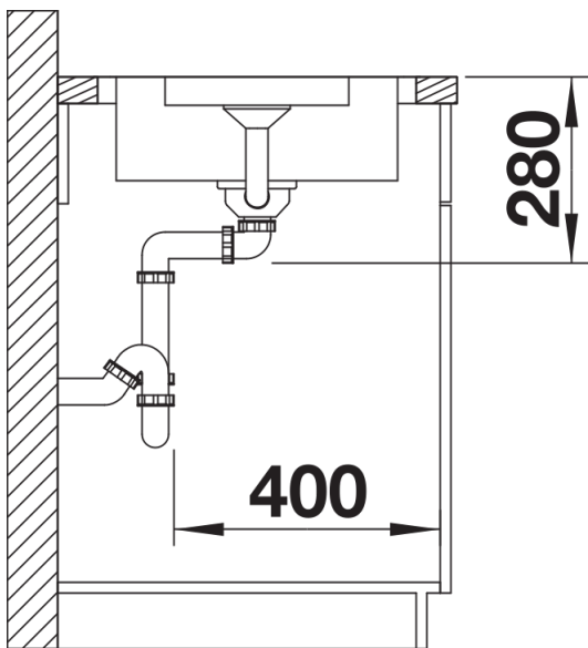
侧视图
