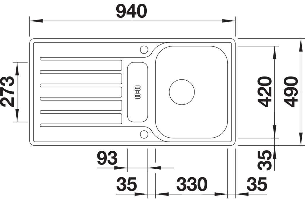
俯视图
