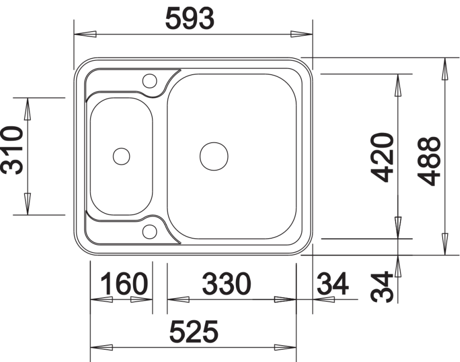
俯视图
