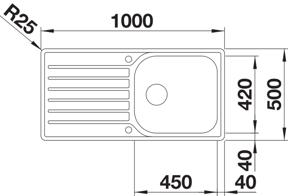
俯视图
