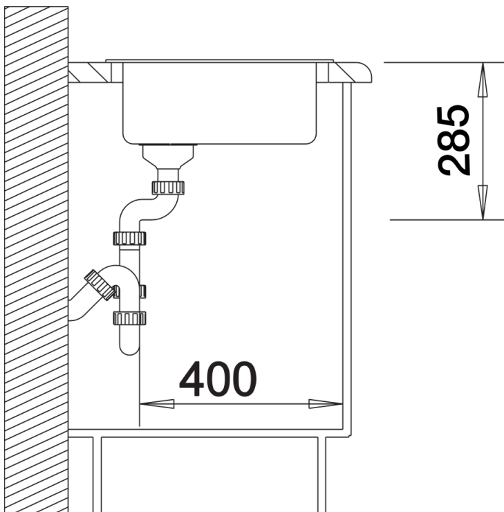
侧视图
