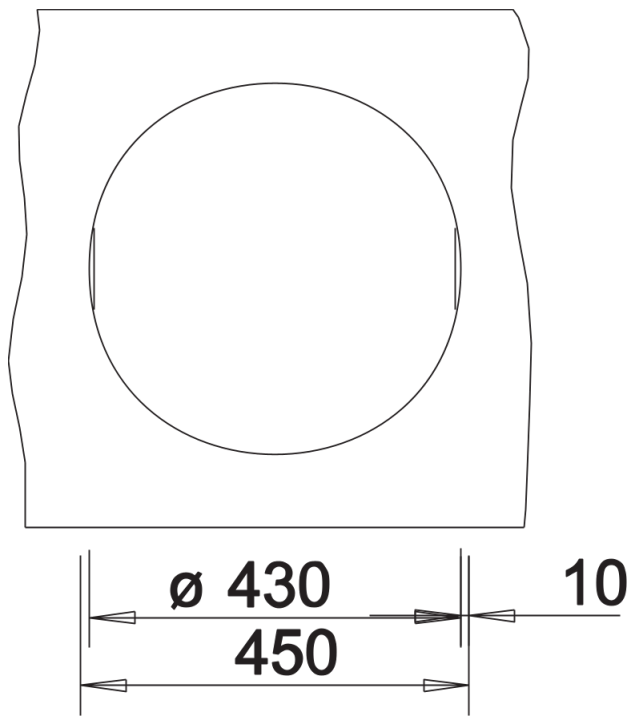
开孔
