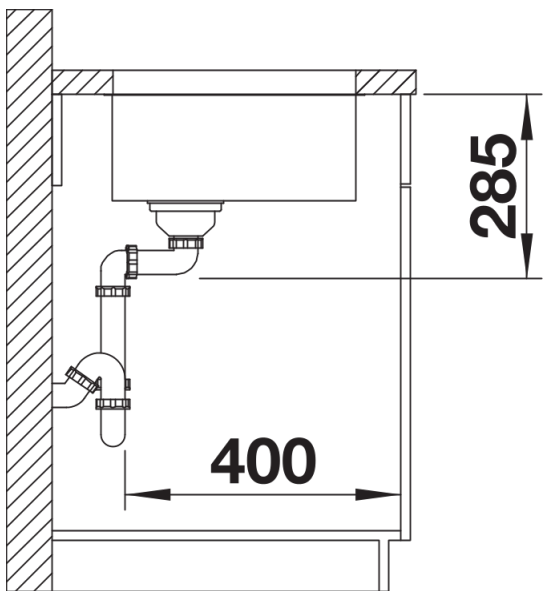
侧视图
