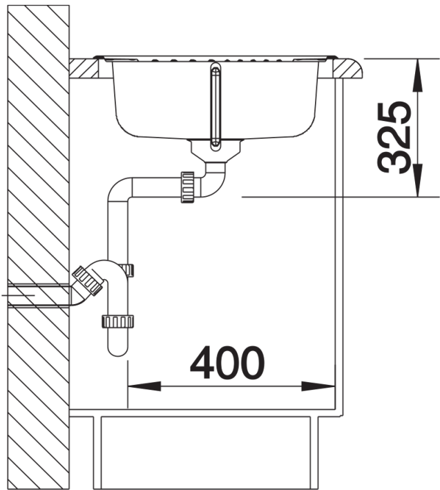
侧视图
