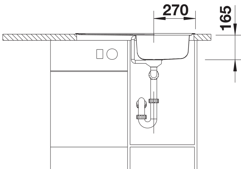
正视图
