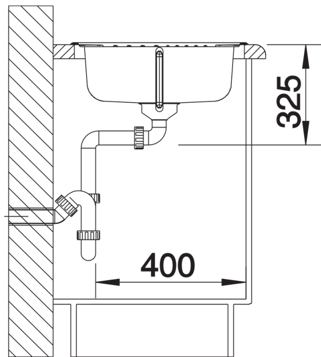
侧视图
