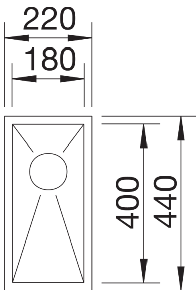
俯视图
