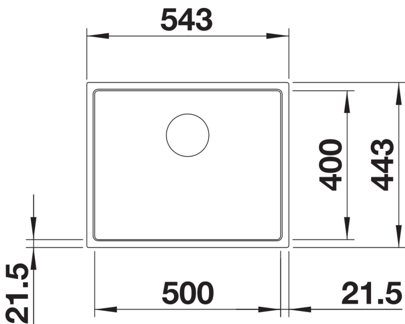
俯视图
