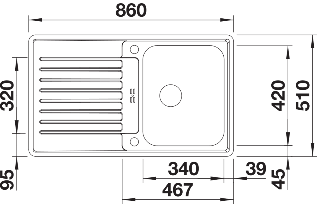
俯视图
