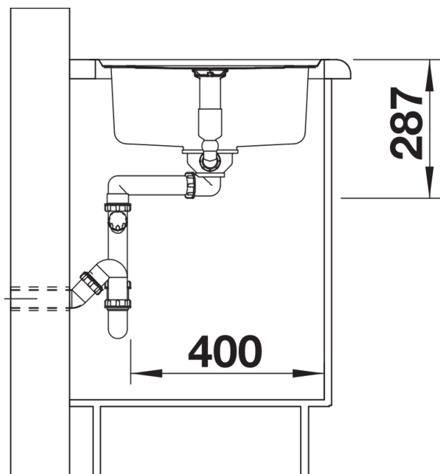
侧视图
