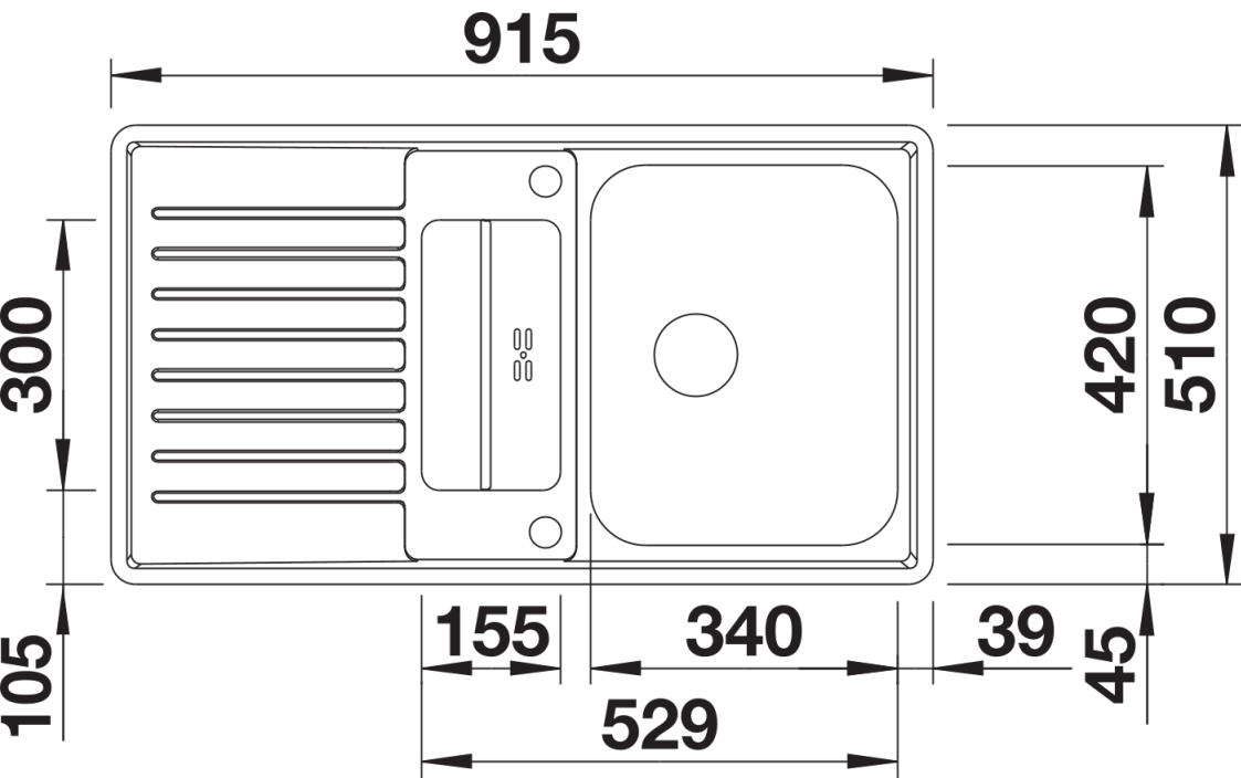
俯视图
