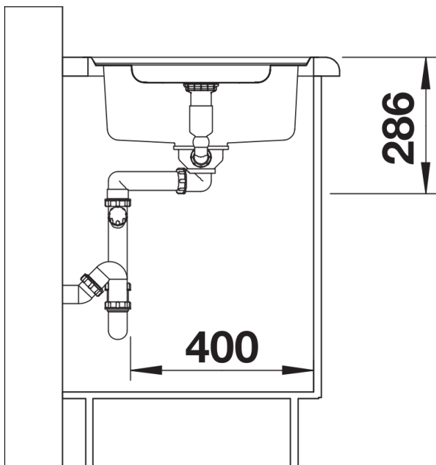
侧视图
