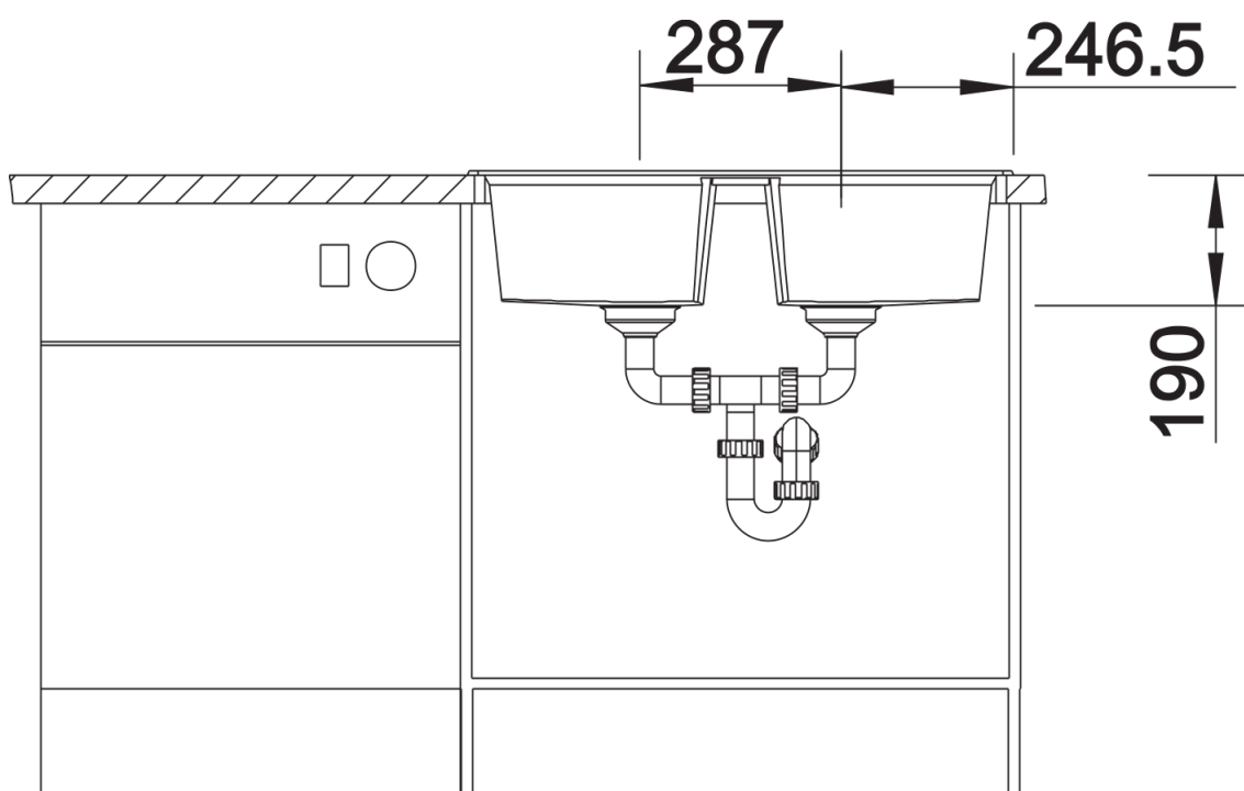
Čelní pohled
