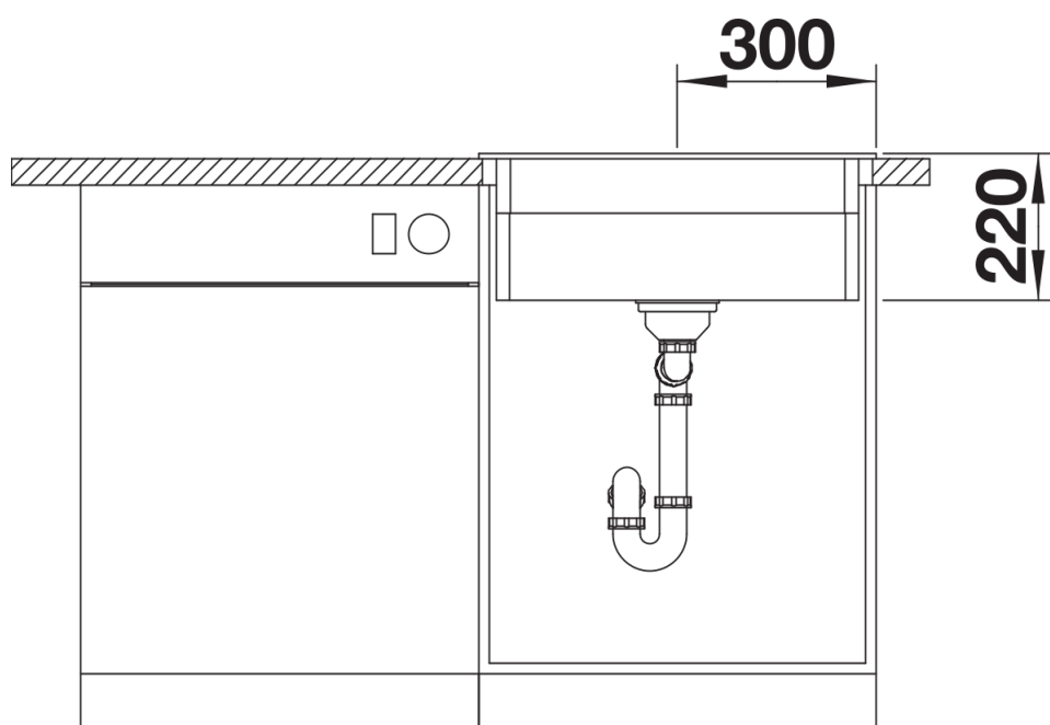
Čelní pohled
