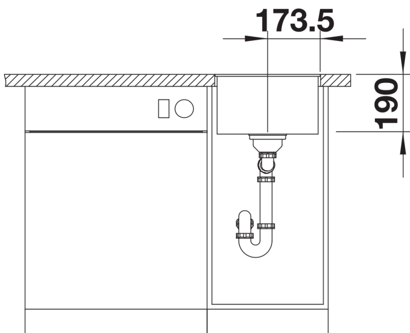
Čelní pohled
