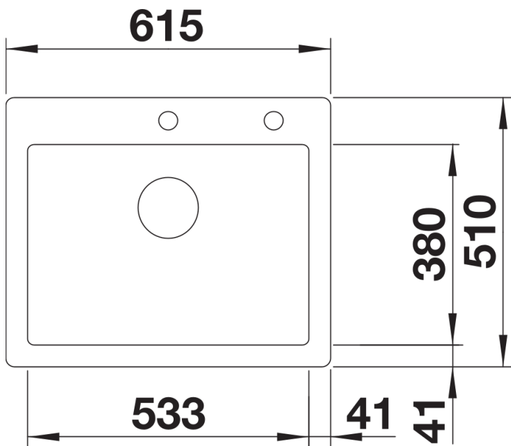
Aufsicht
