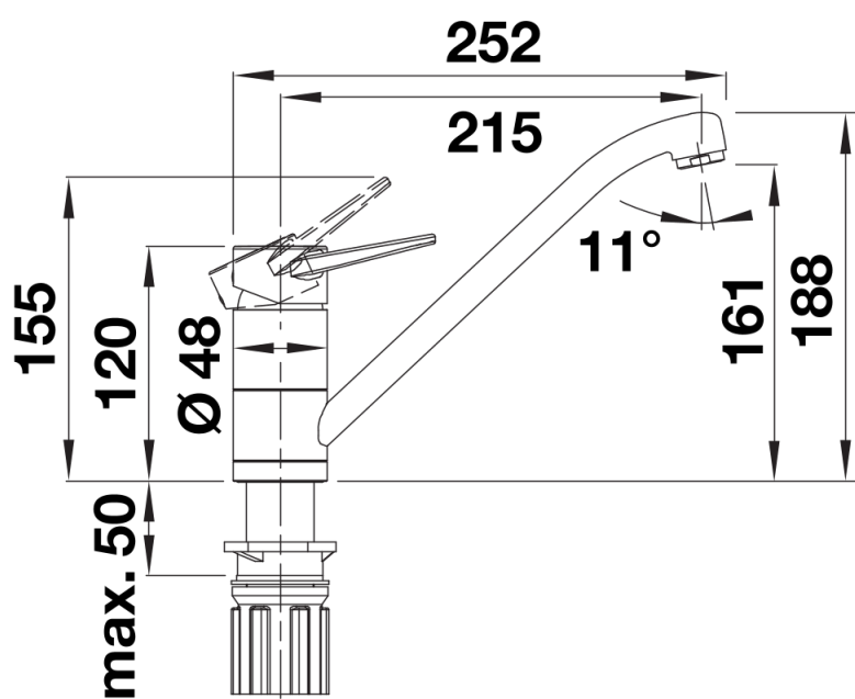
Seitenansicht
