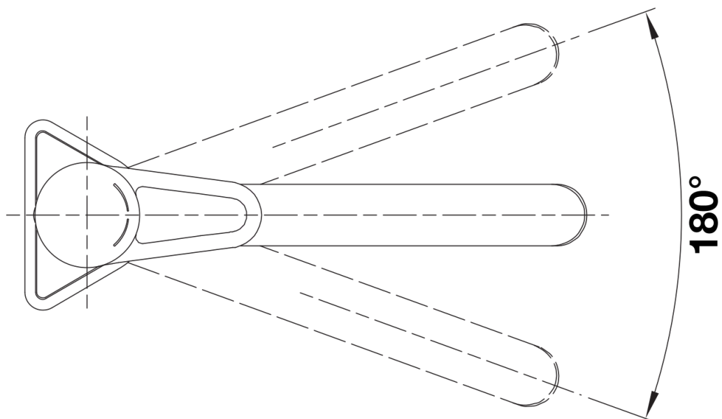
Schwenkbereich
