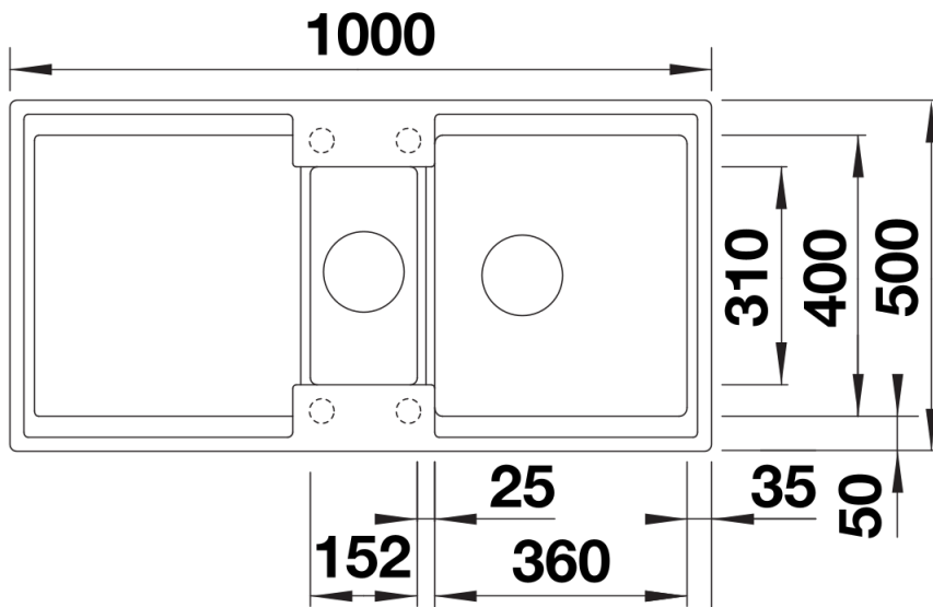
Aufsicht
