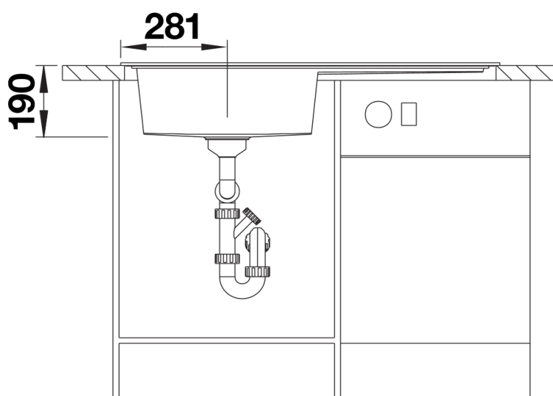
Frontansicht
