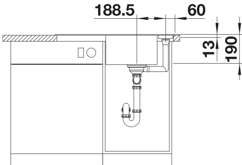
Frontansicht
