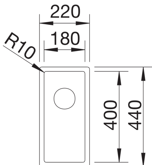
Aufsicht
