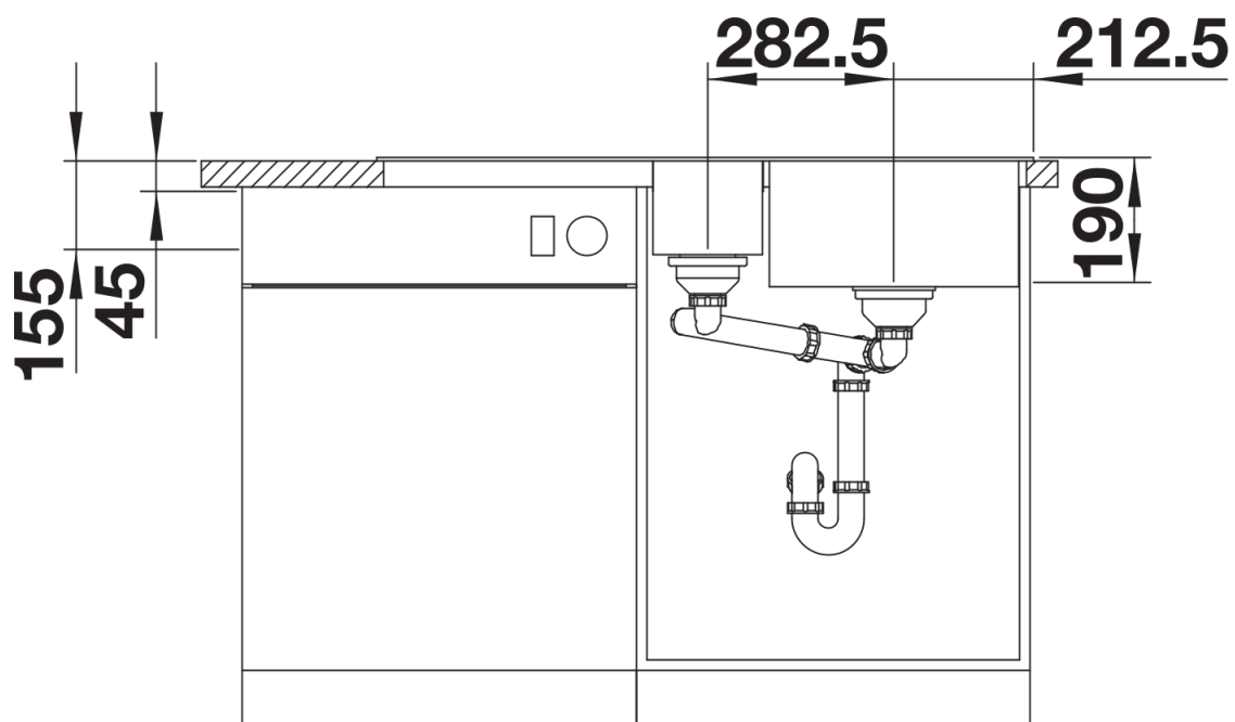
Frontansicht
