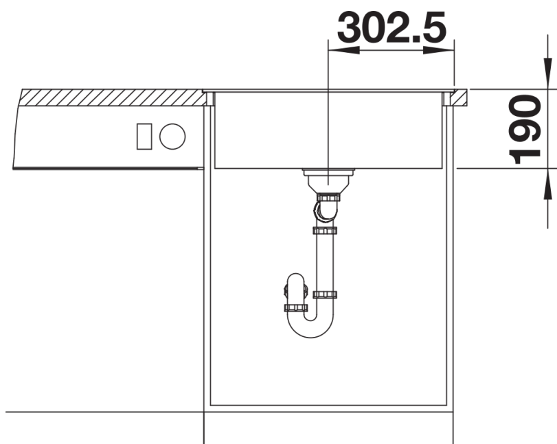
Frontansicht
