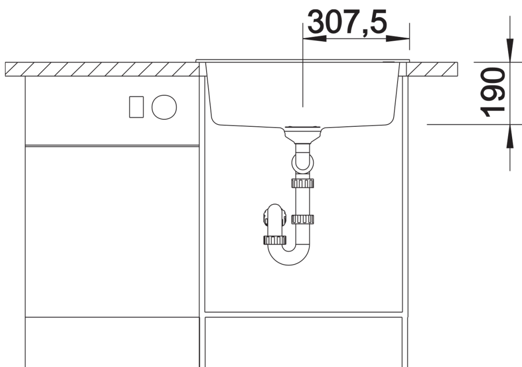
Frontansicht
