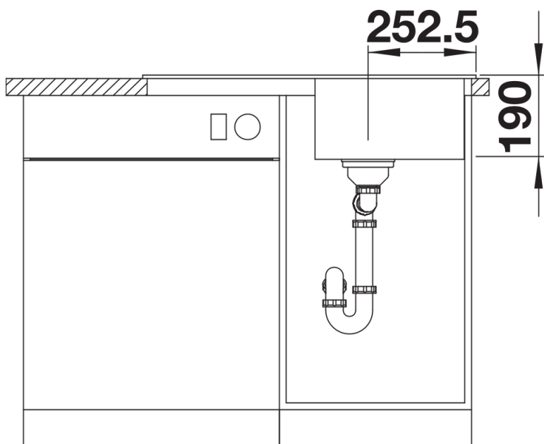
Frontansicht
