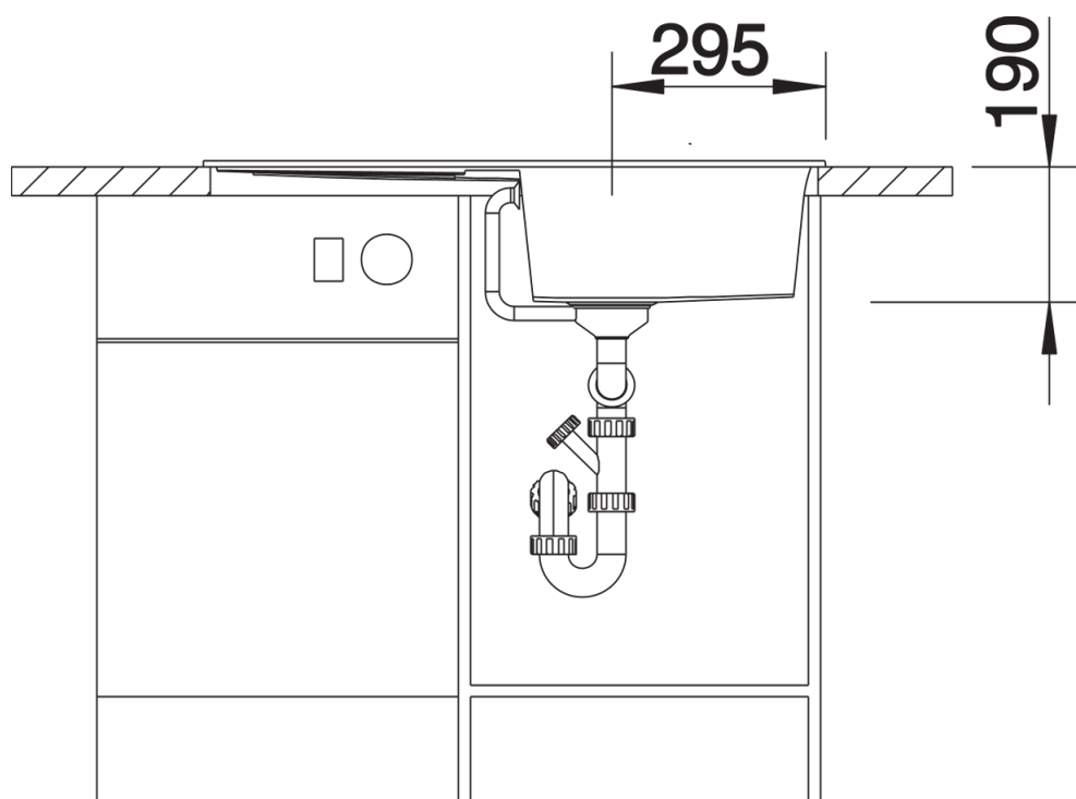
Frontansicht
