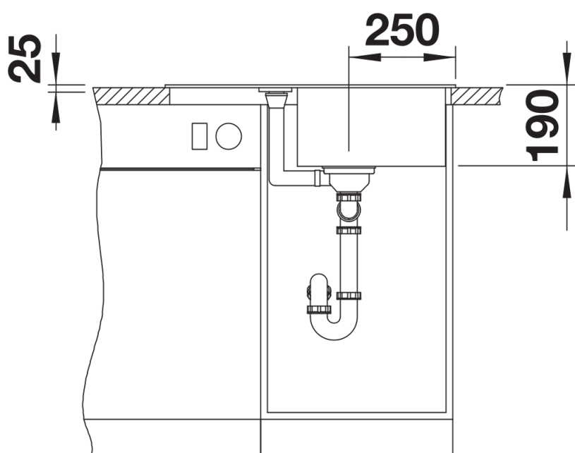
Frontansicht
